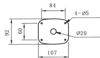
安装平台
