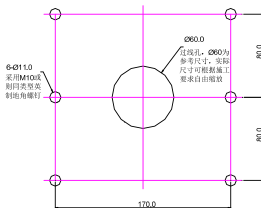
壁装钻攻图
