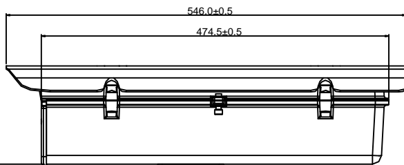
云台正视
