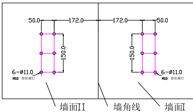
角装适配器钻攻图
