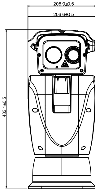
云台正视
