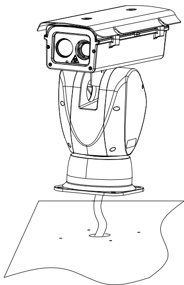
台面安装钻攻图
